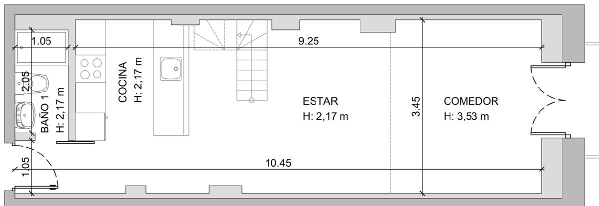
PLANTA BAJA
